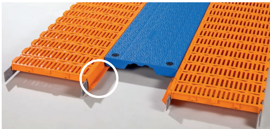
Образец монтажа: простая интеграция плит обогрева за счет несущих реек
